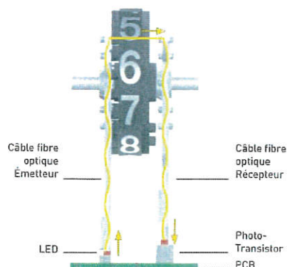
Lecture du nouveau système GWF
