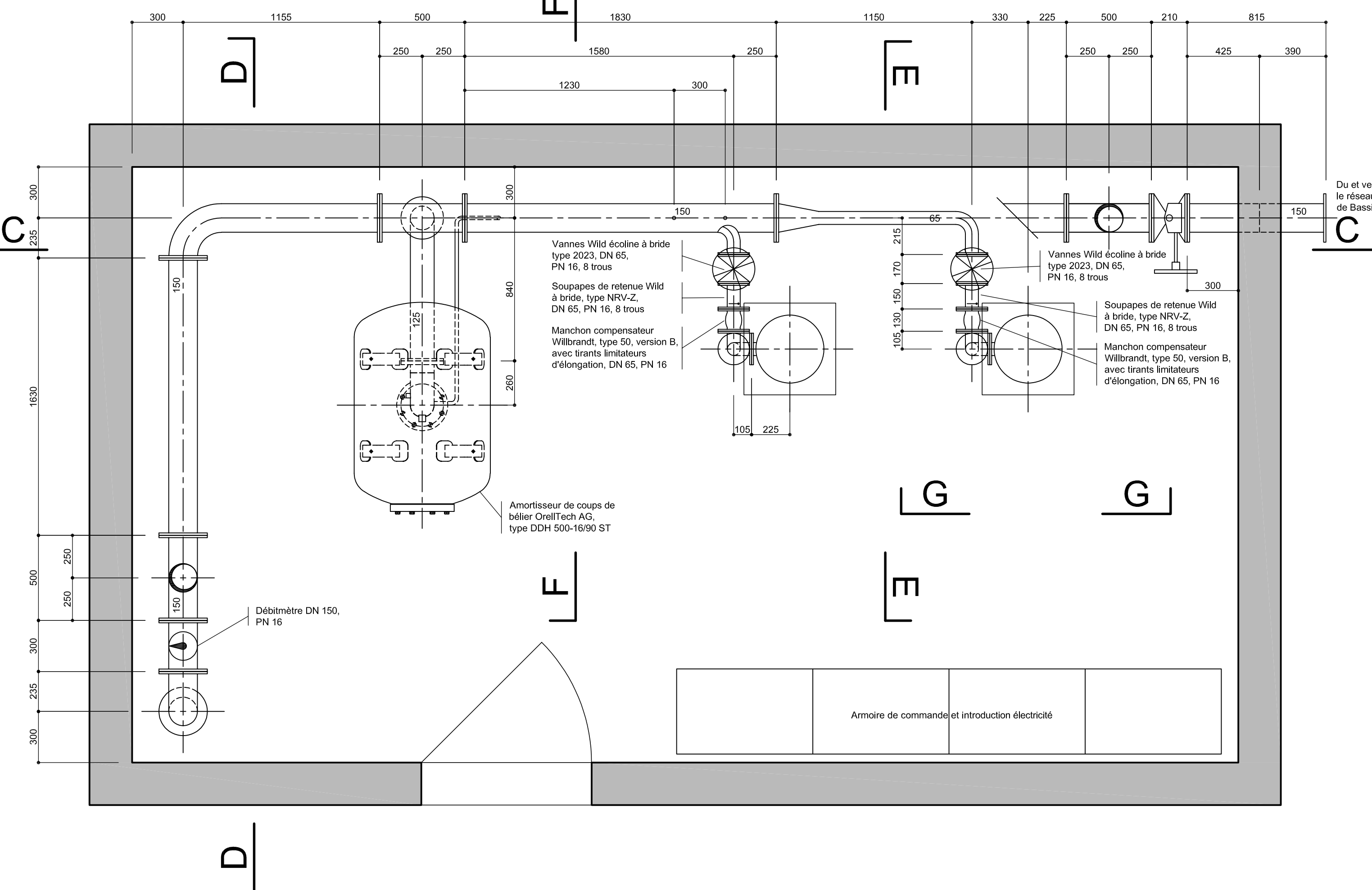
Plan - coupe B - B 1:20
