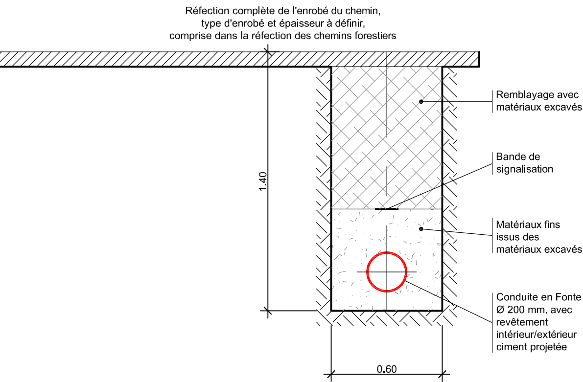
Coupe-type B - B 1:20 Tronçon H - I - J - K - L
